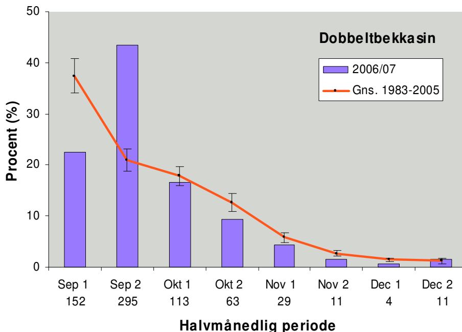
Figur 3. Tidsmæssig fordeling af vinger af dobbeltbekkasin nedlagt i jagtsæsonen 2006/07 og den gennemsnitlige fordeling for perioden 1983/84-2005/06 med 95 % konfidens intervaller.
