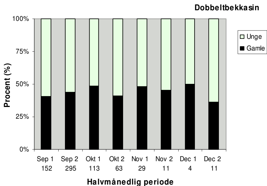
Figur 4. Køns- og alderssammensætning af dobbeltbekkasinvinger gennem jagtsæsonen 2006/07. Antallet af vinger er angivet under søjlerne. Sex and age composition of Snipe wings during the hunting season 2006/07. The number of wings is shown below columns (columns from above: juvenile, adult)
