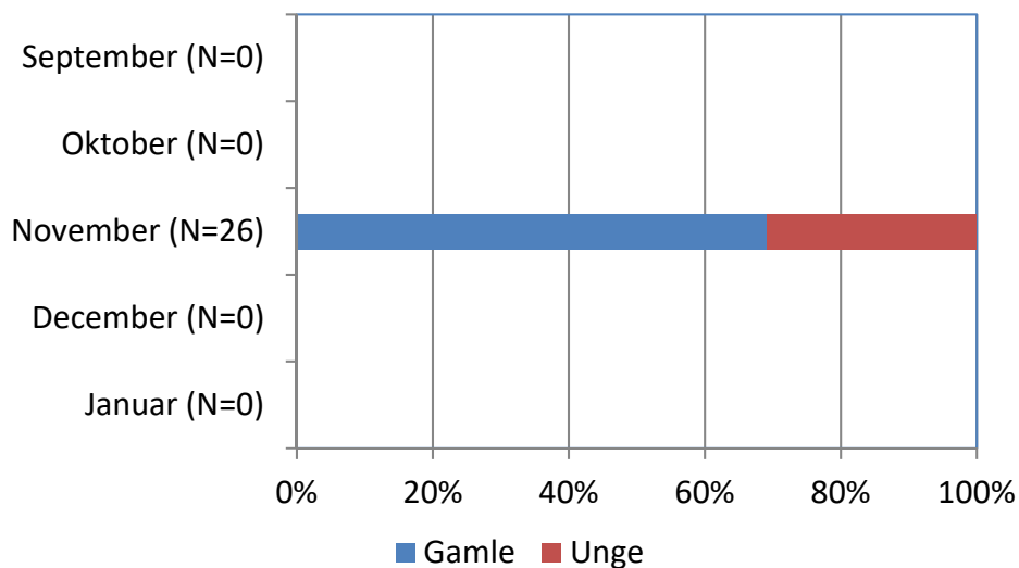
Figur 4. Månedlig fordeling af alderssammensætning af sædgåsevinger gennem jagtsæsonen 2020/21. Antallet af vinger er angivet. The monthly age composition of Bean Goose wings during the hunting season 2020/21 (rows from the left: adults and juveniles). The number of wings is shown.
