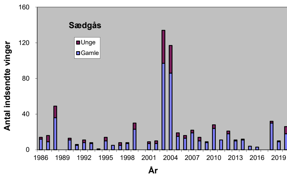
Figur 2. Antallet af indsendte vinger af sædgås fra jagtsæsonerne 1986/87-2020/21. The number of Bean Goose wings received from the hunting seasons 1986/87-2020/21.
