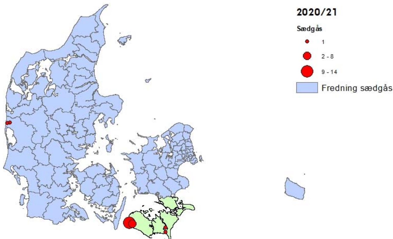
Figur 1. Geografisk fordeling af 26 vinger af sædgås indsendt gennem jagtsæsonen 2020/21.
