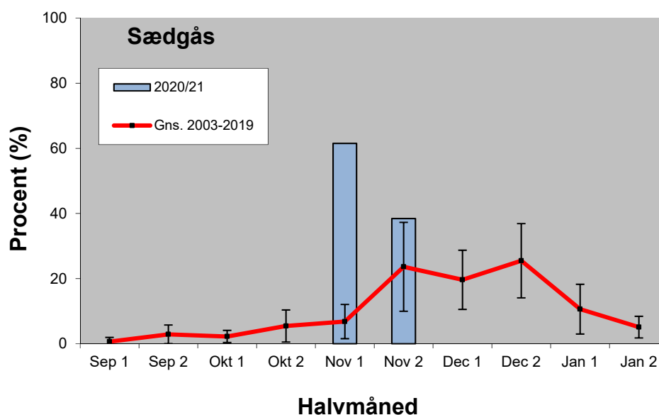
Figur 3. Tidsmæssig fordeling af vinger af sædgås nedlagt i jagtsæsonen 2020/21 og den gennemsnitlige fordeling for perioden 2003/04-2019/20 med 95 % konfidensintervaller. Temporal distribution of wings from Bean Goose bagged during the 2020/21 hunting season and the mean and 95% confidence intervals of the period 2003/04-2019/20.
