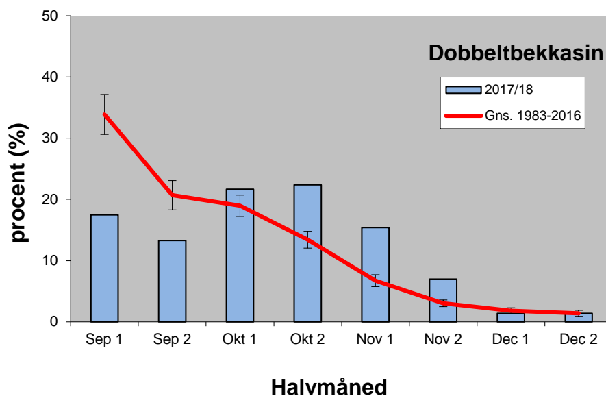
Figur 3. Tidsmæssig fordeling af vinger af dobbeltbekkasin nedlagt i jagtsæsonen 2017/18 og den gennemsnitlige fordeling for perioden 1983/84-2015/16 med 95 % konfidens intervaller.
